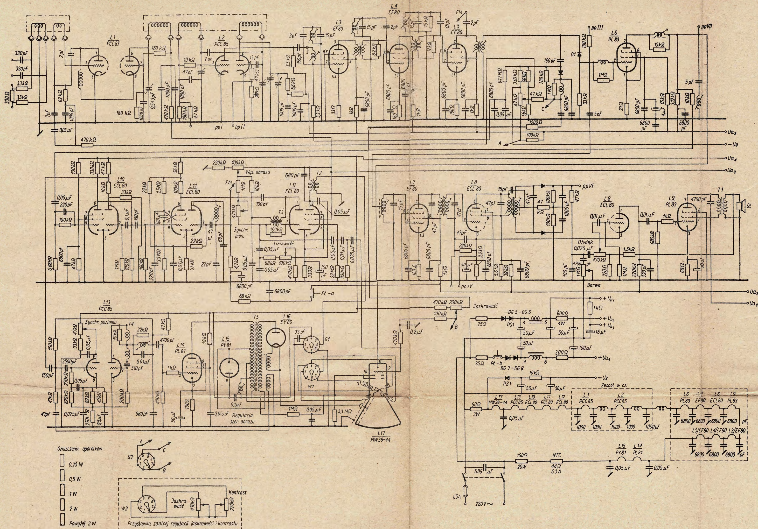
Rys. 10-22. Schemat ideowy odbiornika Belweder I
