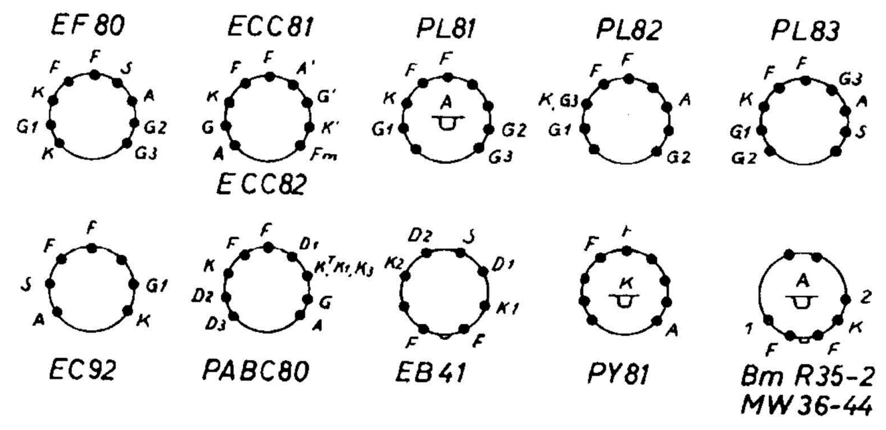
Schaltschema SABA-Schauinsland WII 5291 F565
