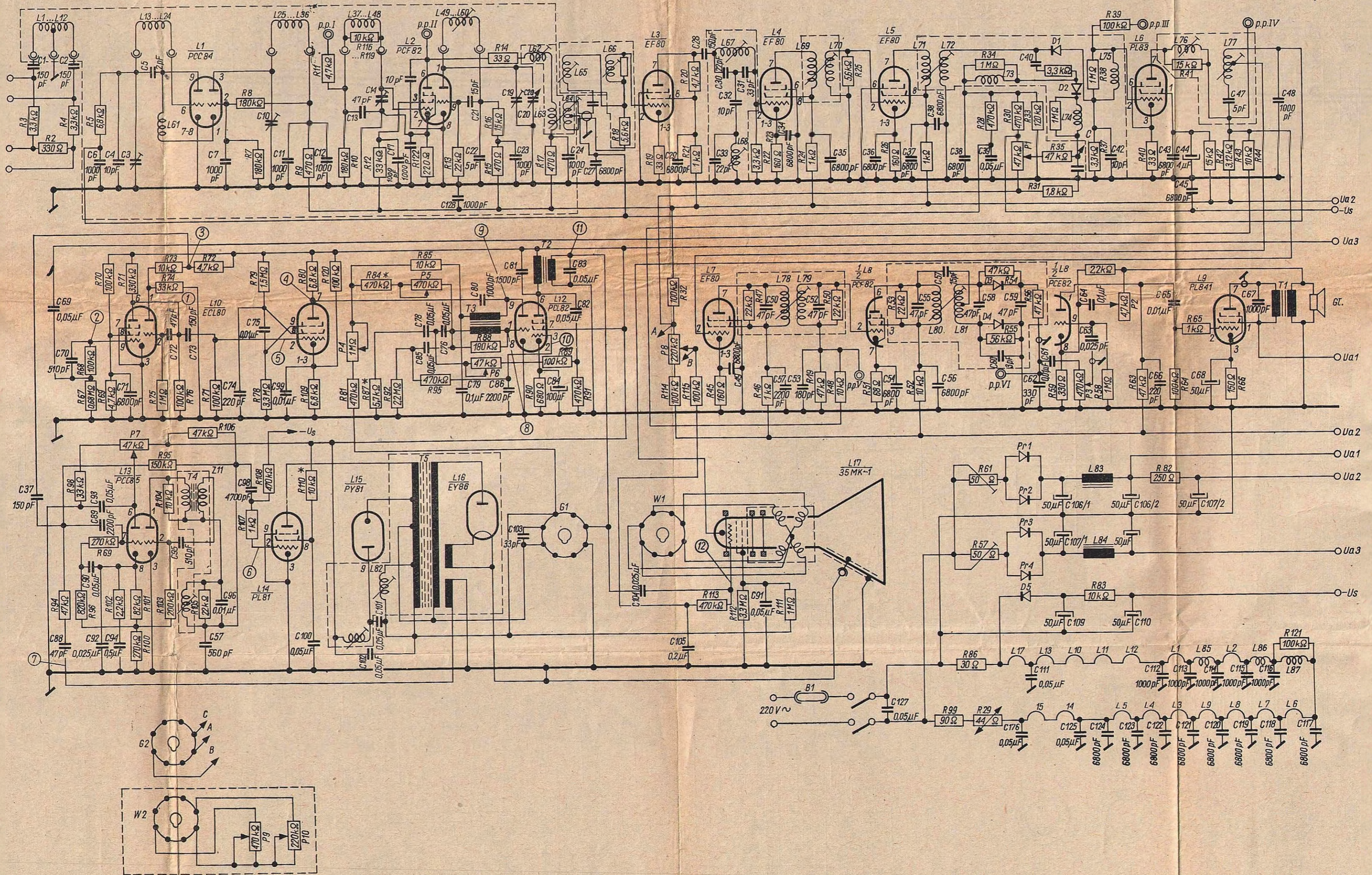
Rys. 10-64. Schemat ideowy odbiornika Turkus OT 1491
