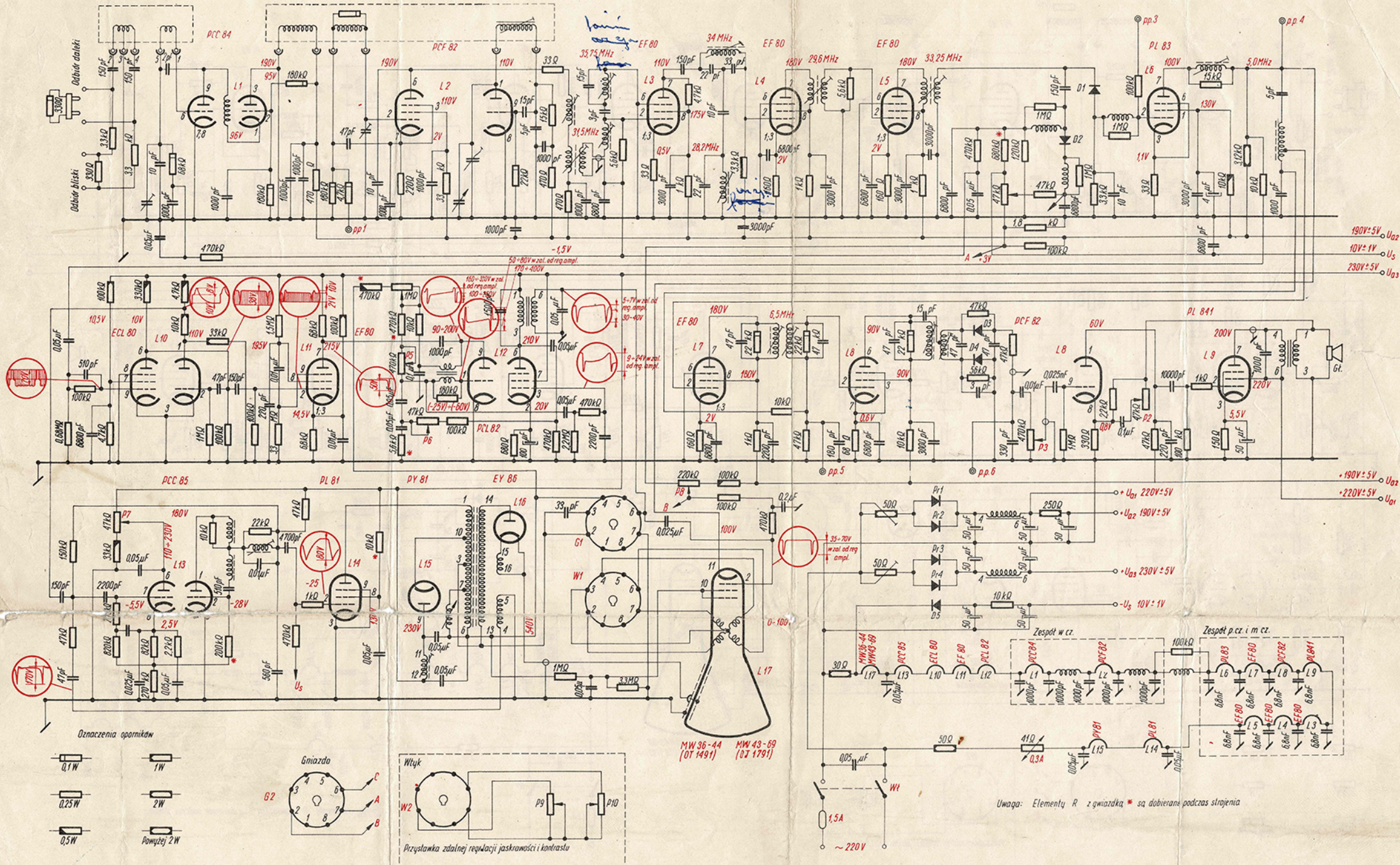
Schemat 1. Odbiornik telewizyjny Turkus (Jantar i Smaragd)
