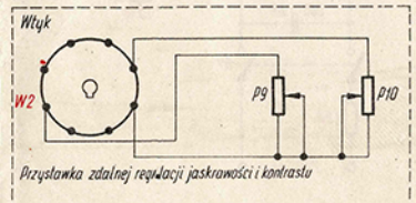
Schemat 1. Odbiornik telewizyjny Turkus (Jantar i Smaragd)
