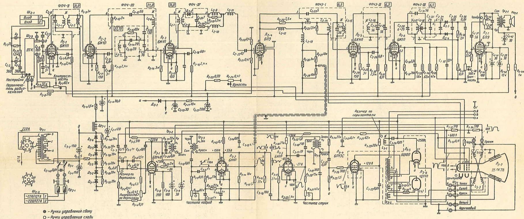
Принципиальная схема телевизора «Рекорд-12»
