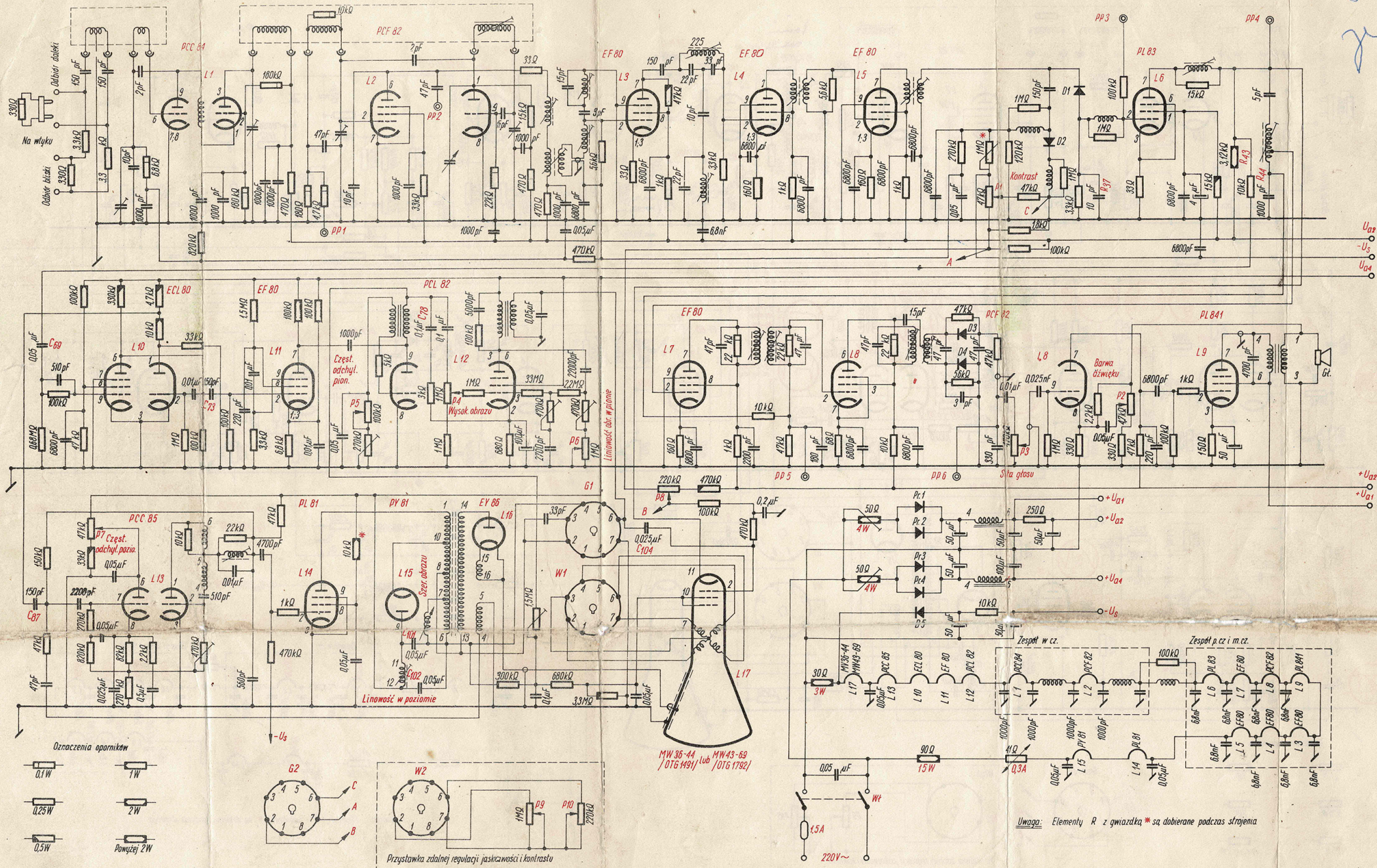
Schemat 2. Odbornik telewizyjny Neptun
